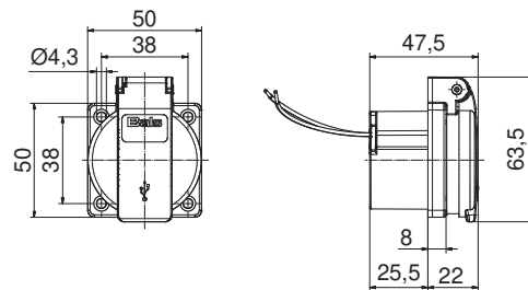
Einbauöffnung
